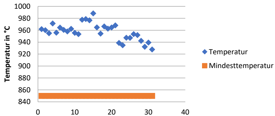
Verbrennungsbedingungen - Januar 2019
