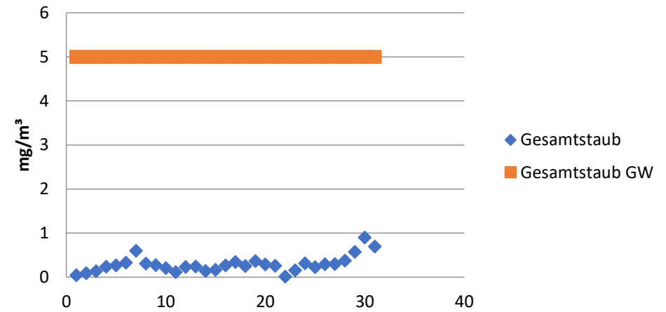
Gesamtstaub - Januar 2019
