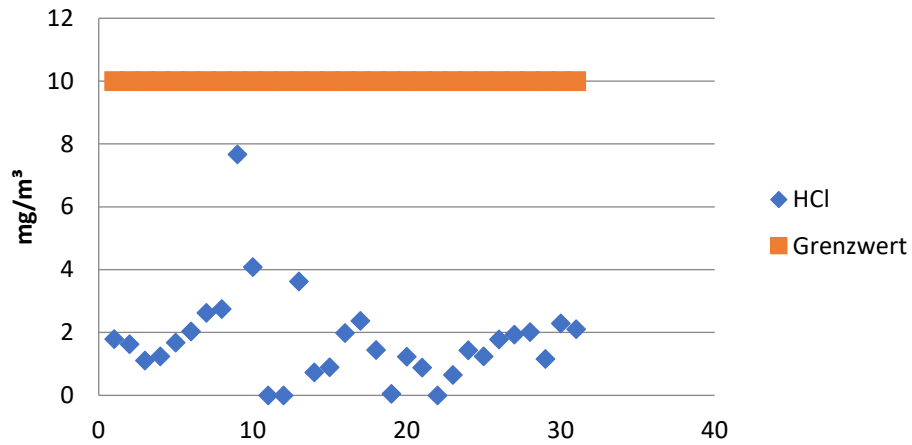
HCl - Januar 2019
